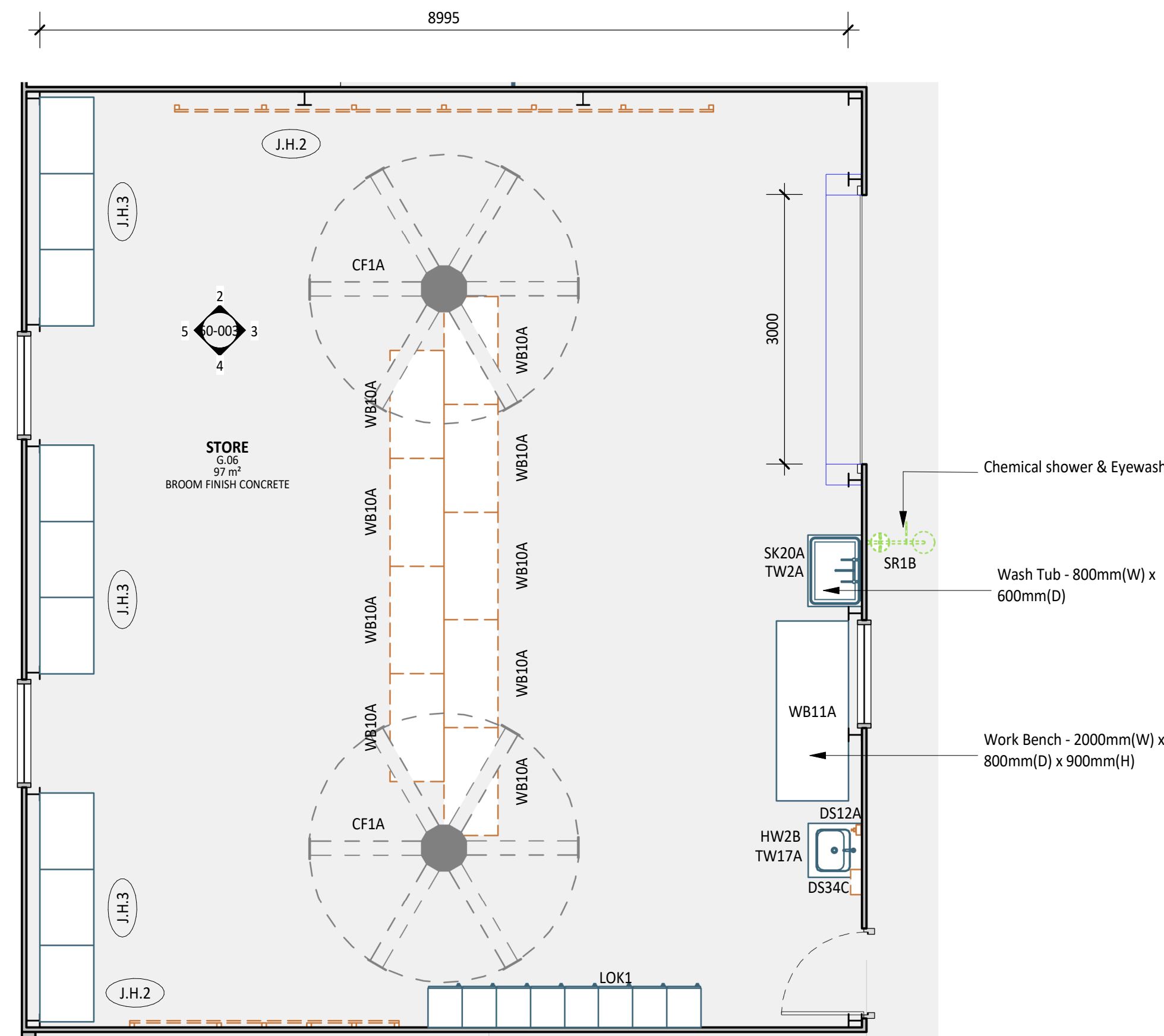
1 PLAN DETAIL 1 : 50
